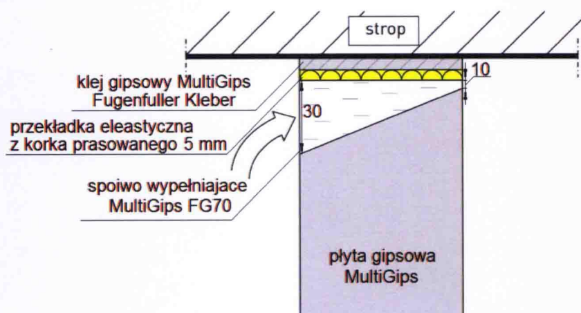
Rys. 3. Schemat połączenia ściany z płyt gipsowych ze stropem.
