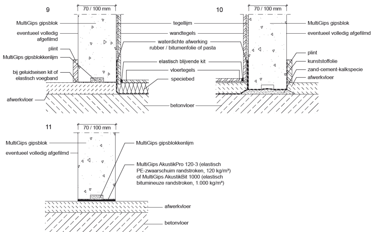
VLOERAANSLUITINGEN (6: ruwe vloer; 7: afgewerkte vloer; 8 – 10: vloer in natte ruimte; 11: met elastische randstroken)
