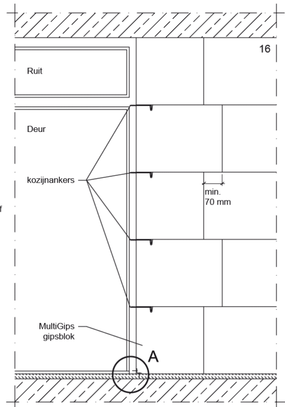
AANSLUITING KOZIJSIJL
