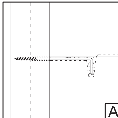
detail: kozijnanker
